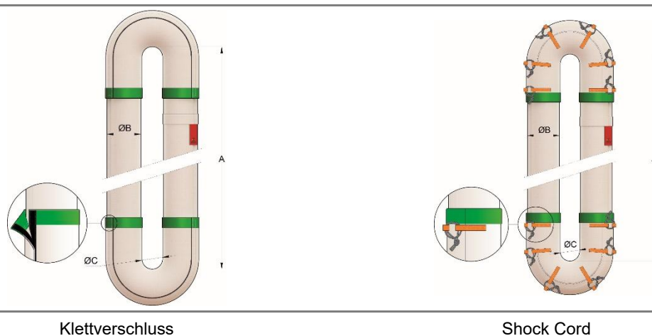
Abbildung 14: Verschleißpads
